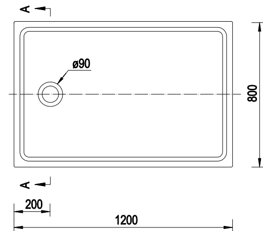
PURE 120x80x3,5 cm (EMPORIA-PURE0006)
