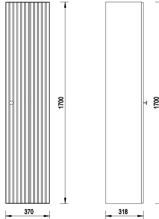
RIO 37 37x31,8x170 cm (EMPORIA-001-C-03702 | EMPORIA-001-C-03703)
